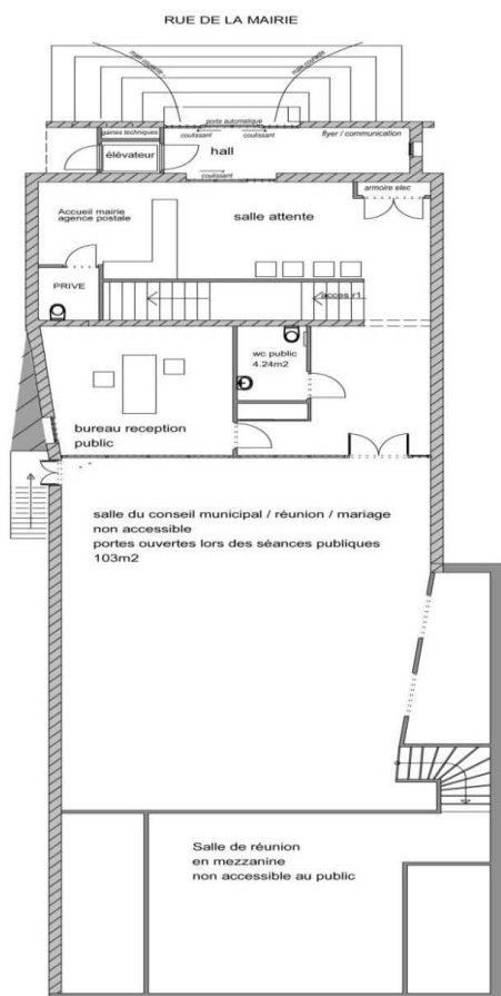
↑ PLAN DU REAMENAGEMENT DE LA MAIRIE
